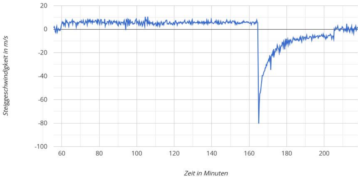
Zeit / Steiggeschwindigkeit
