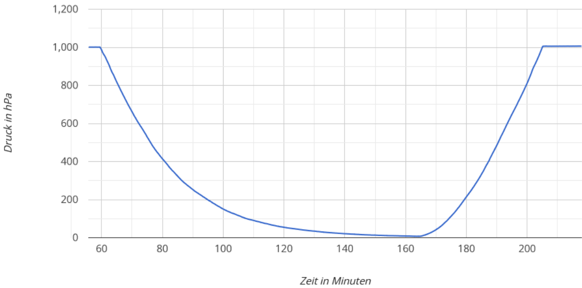
Zeit / Druck
