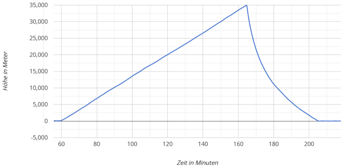
Zeit / Höhe
